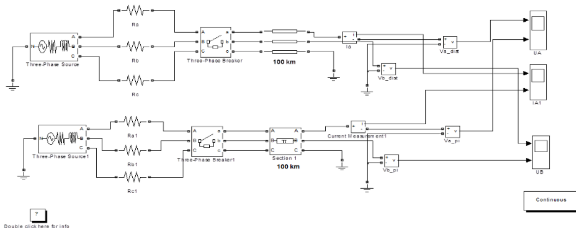
Рисунок 1 – Имитационные модели ЛЭП 110 кВ длиной 100 км с распределенными параметрами и с сосредоточенными параметрами
