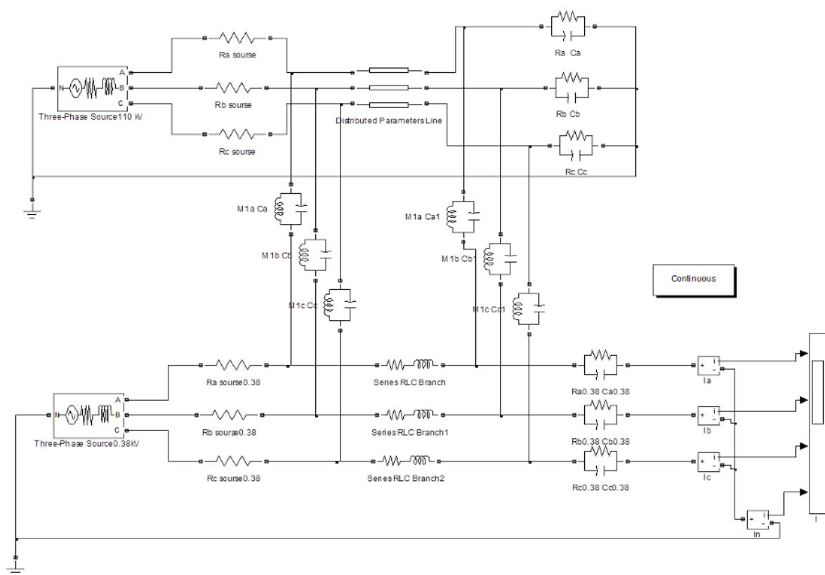
Рисунок 2 – Имитационная модель влияния ВЛЭП 110 кВ на ЛЭП 0,38кВ
