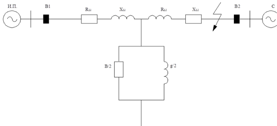
Рисунок 1 – Однолинейная электрическая схема замещения трехфазной линии электропередач напряжением 110 кВ с однофазным коротким замыканием
