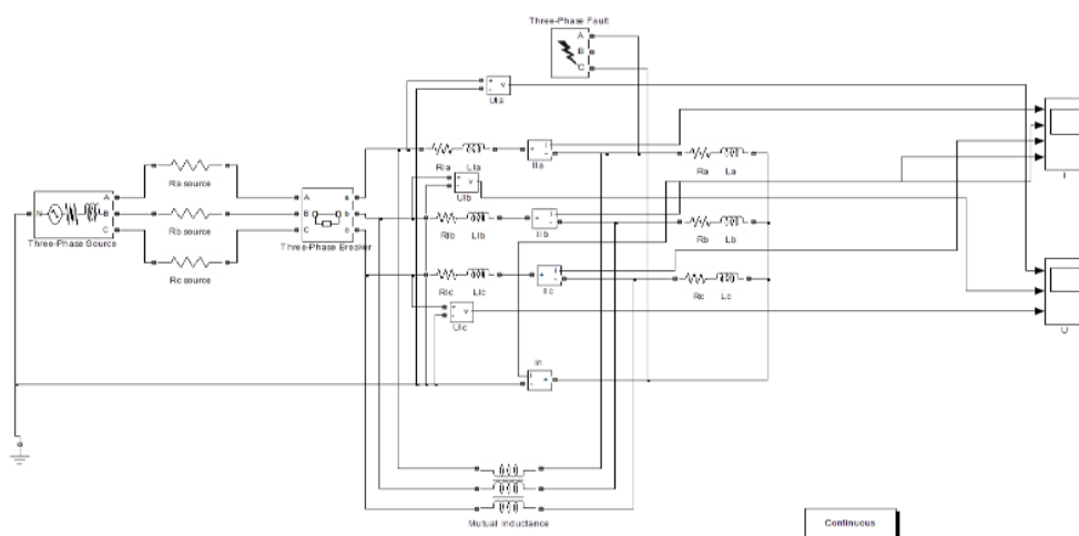
Рисунок 2 – Имитационная модель линии электропередач напряжением 110 кВ, соответствующая принципиальной схеме замещения с однофазным коротким замыканием.
