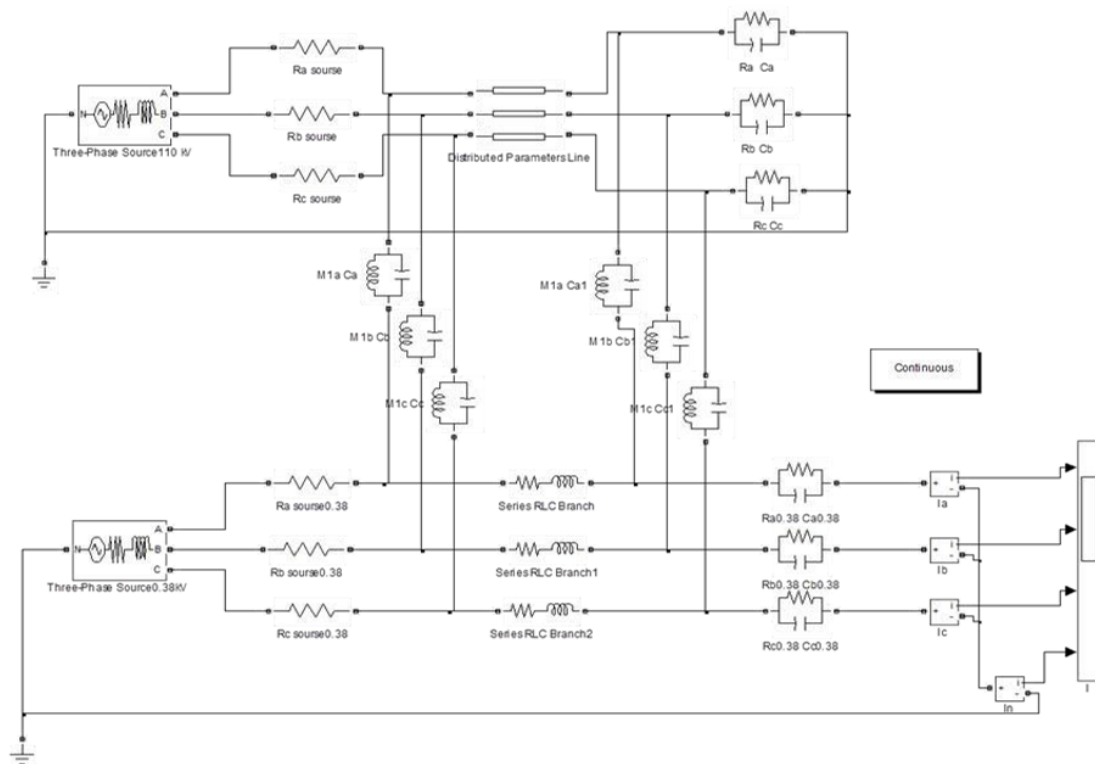
Рисунок 2 – Имитационная модель влияния ВЛЭП 110 кВ на ЛЭП 0,38кВ Анализ коэффициентов несинусоидальности кривой тока.
