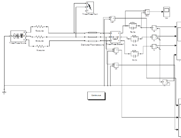
Рисунок 1 – Имитационная модель ЛЭП 110 кВ длиной 100 км при двухфазном коротком замыканием.
