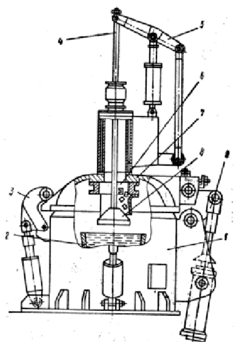
Рис. 1 – Камера-автоклав для введения магния в расплав чугуна
