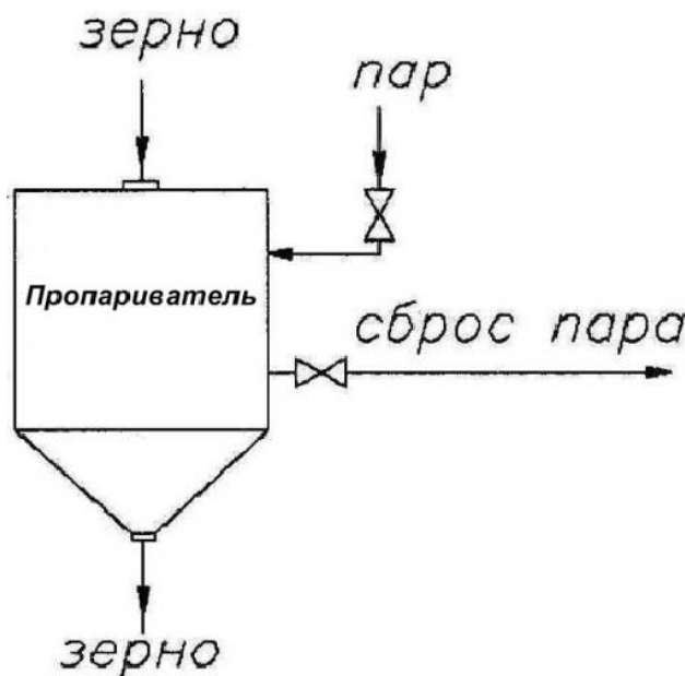
Рисунок 7.14 – Пропаривание зерна
