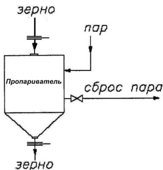
Рисунок 7.13 – Пропаривание зерна (на крупозаводе)
