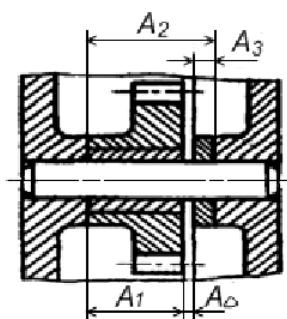
Рис. 1. Размерная цепь, обеспечивающая зазор A_4
