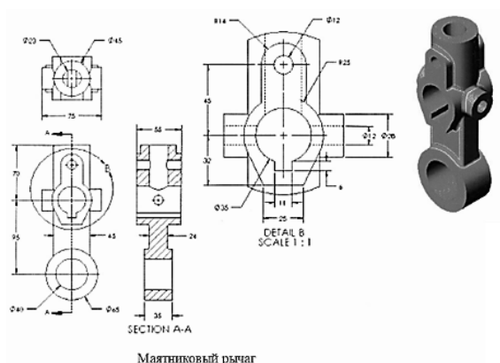
Маятниковый рычаг
