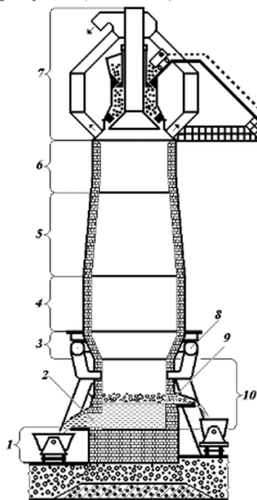
Рисунок – Доменная печь
