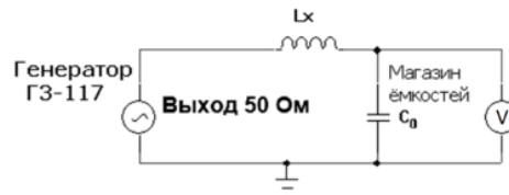
Рисунок – Принципиальная схема для измерения индуктивности
