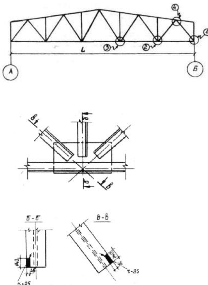
Схема стропильной фермы
