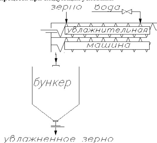
Рисунок 7.16 – Увлажнение зерна
