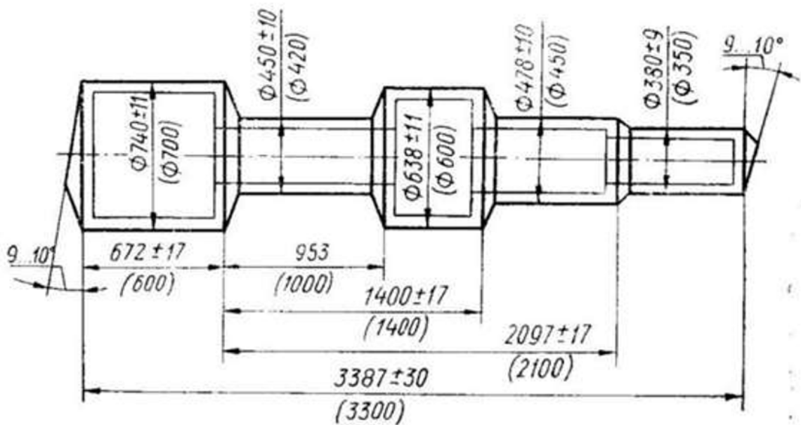
Чертеж заготовки
